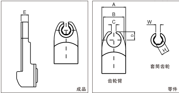
成品齿轮臂外形尺寸
