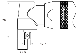
头部尺寸参考图:
