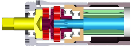
结构示意图：
