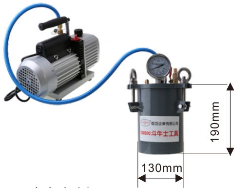
真空注油机
