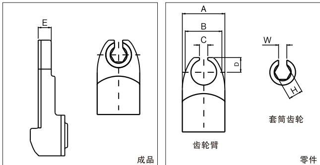
成品齿轮臂外形尺寸
