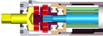
结构示意图：
